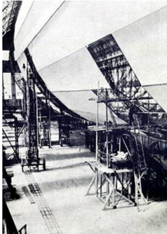
Proceso de entelado y construcción de una de las góndolas que albergaba los poderosos motores Maybach del LZ 127. Fuente: Colección CLA.
