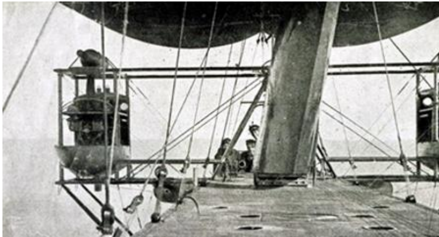
Vista posterior de la cabina, góndolas motrices y la típica envuelta trilobulada de un dirigible Astra-Torres. Fuente: Colección CLA.
