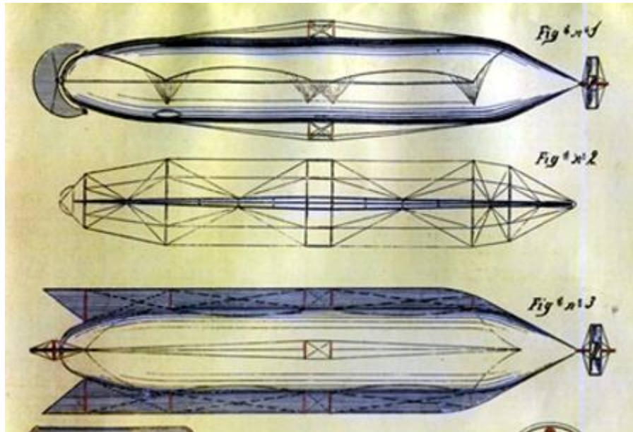
Plano del dirigible del español Ricardo Fradera en el que se muestra su complicada estructura presidida por el estabilizador longitudinal. Fuente:
